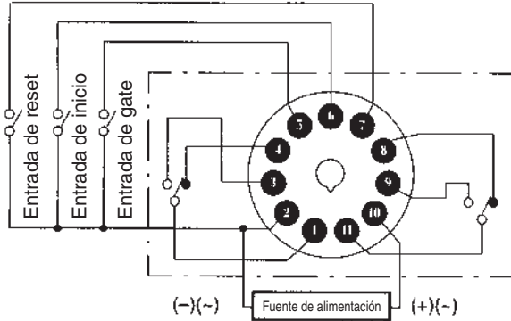
H3CR-AS (Salida de transistor)
