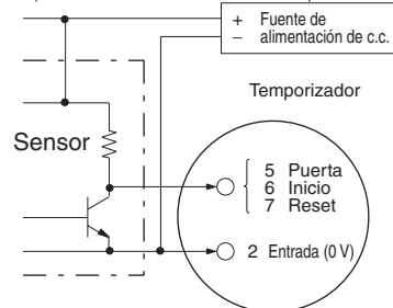
Funciona con transistor en ON
