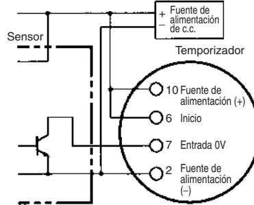
Funciona con transistor NPN en ON
