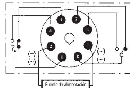
H3CR-A8E (Salida de contacto)
