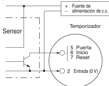
Funciona con transistor en ON
