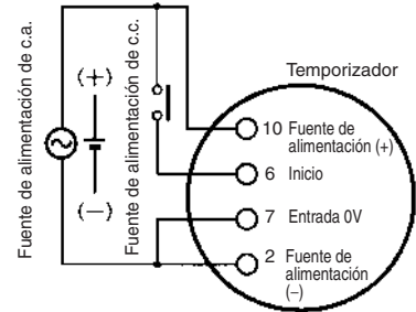
Funciona con relé en ON
