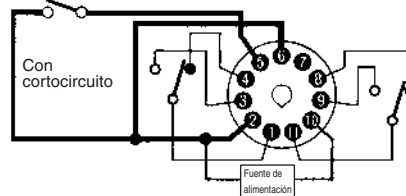
Señal de puerta (el funcionamiento se interrumpe con la señal de puerta si el temporizador detecta una señal anormal)
