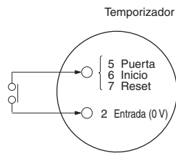
Funciona con relé en ON
