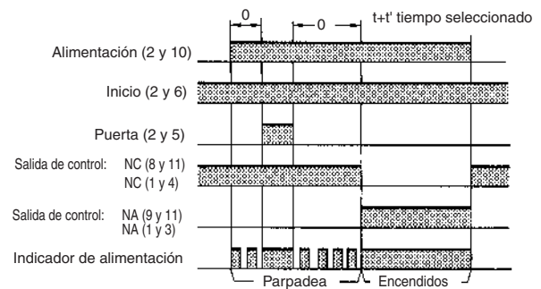
Señal de puerta (el funcionamiento se interrumpe con la señal de puerta si el temporizador detecta una señal anormal)
