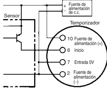
Funciona con transistor PNP en ON
